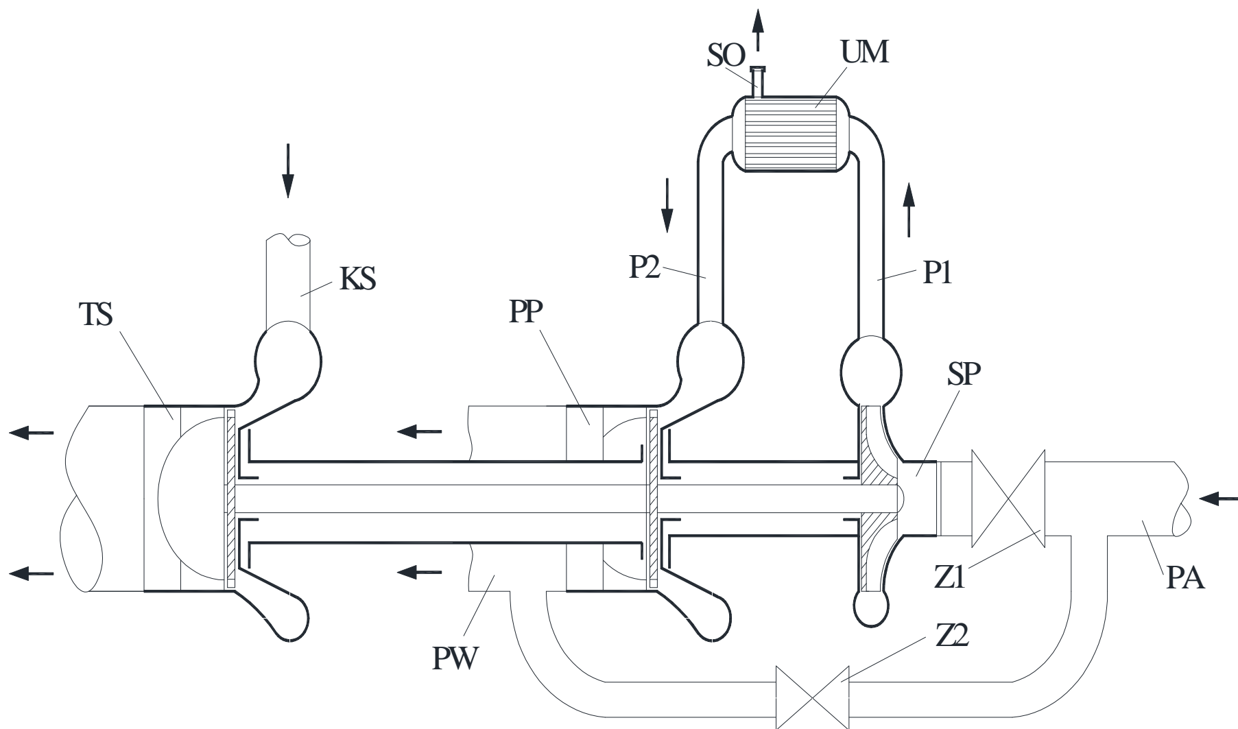
Rys. 1. Schemat turbosprężarkowego układu membranowego do rozdzielu powietrza; PA - przewód wlotowy, SP - sprężarka, TS - turbina spalinowa, P1 - przewód wejściowy, UM - układ membranowy, SO - przewód wylotowy azotu, P2 - przewód wyjściowy, Z1 - wlotowy zawór sterujący, Z2 - zawór sterujący, PW - przewód wylotowy, KS - króciec spalin, PP - pompa próżniowa.
